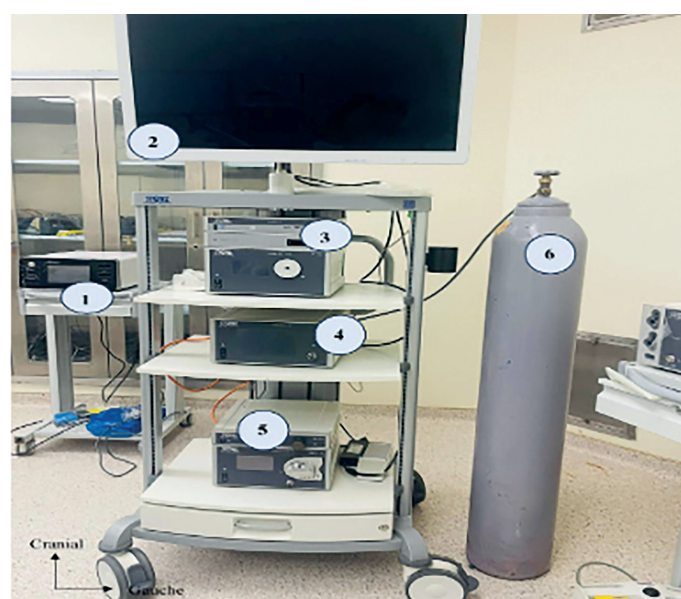
Figure 1 : Colonne complète de laparoscopie.
